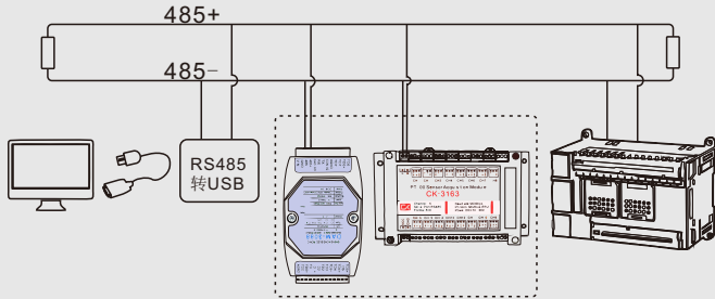
DAM模块通过RS485接口与其它设备组网连接示意图
