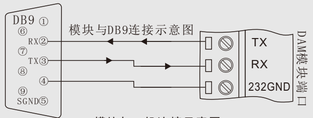
DAM模块与PC机连接示意图
