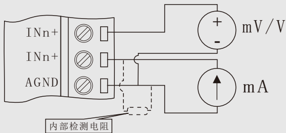
DAM-6160模拟量输入接线示意图
