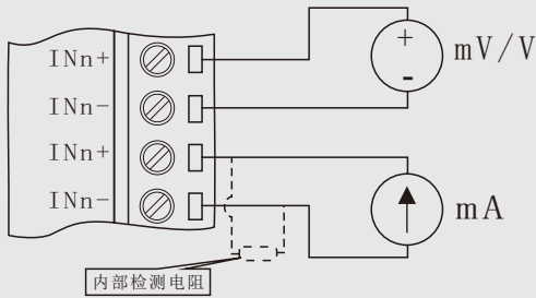
CK-8160E模拟量输入接线示意图
